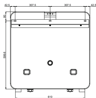
Pohled zezadu
