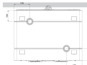
Pohled zdola
