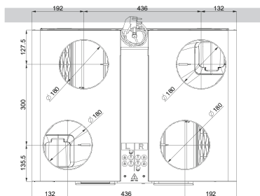
Pohled shora
