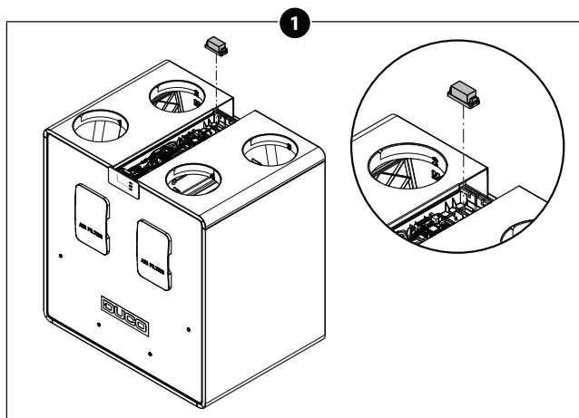
D400 a varianty Plus: Vyjměte transformátor z rozvodné krabice a umístěte jej přímo na určené místo na desce plošných spojů
