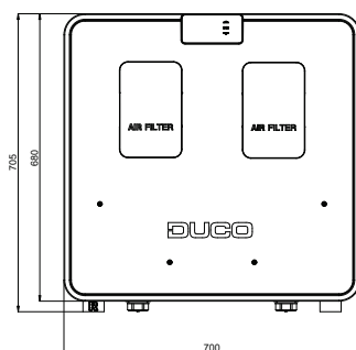
Pohled zepředu
