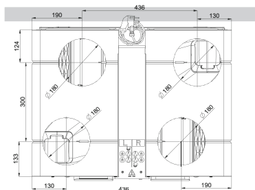
Pohled shora
