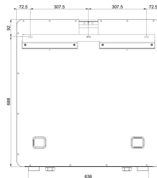
Pohled zezadu
