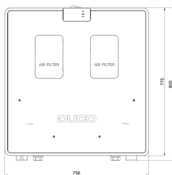
Pohled shora
