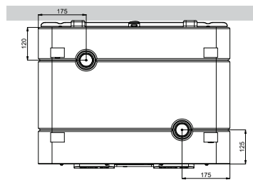
Pohled zdola
