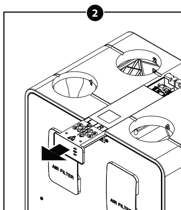
Posuňte kryt dopředu.
