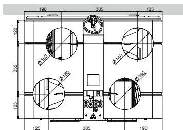
Pohled shora
