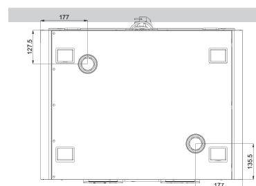
Pohled zdola
