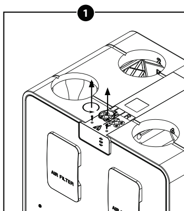
Povolte šrouby.
