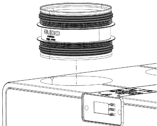
Zatlačte připojovací objímku do jednotky
